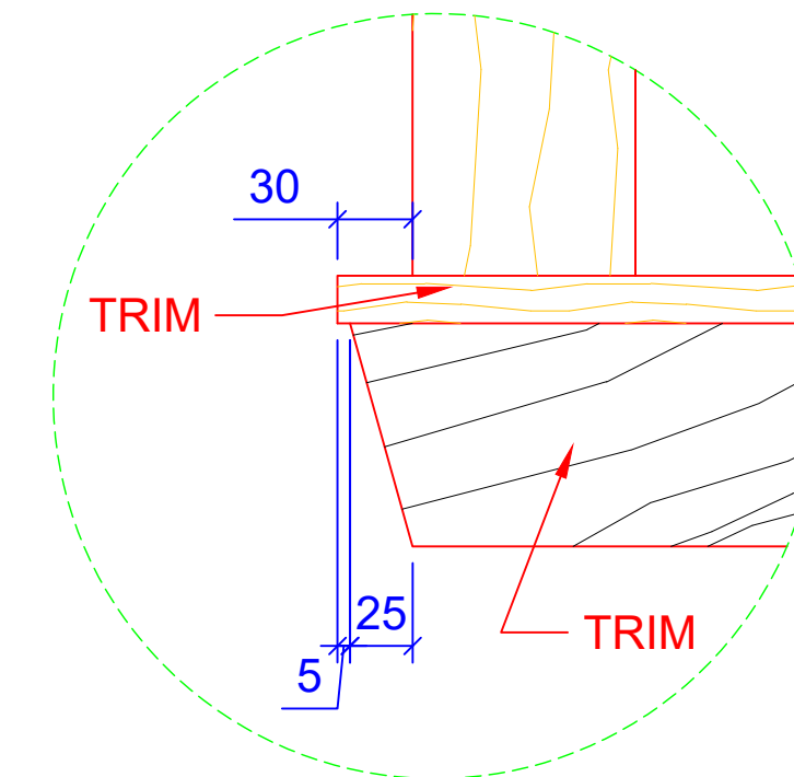
7 WINDOW SILL TRIM A4
