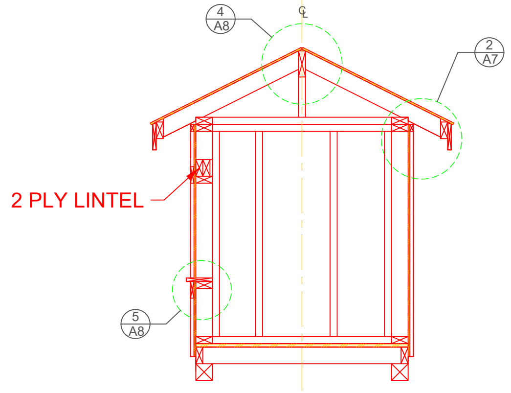
SECTION-A A2, A3, A4, A5
