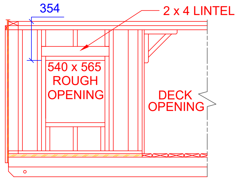
SECTION-C A2
