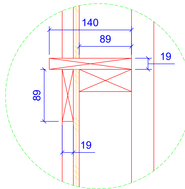
5 WINDOW SILL A6
