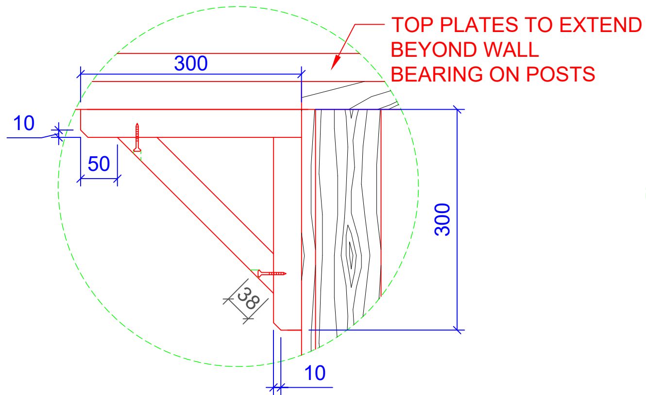
9 BRACE DETAIL-SIDE A5
