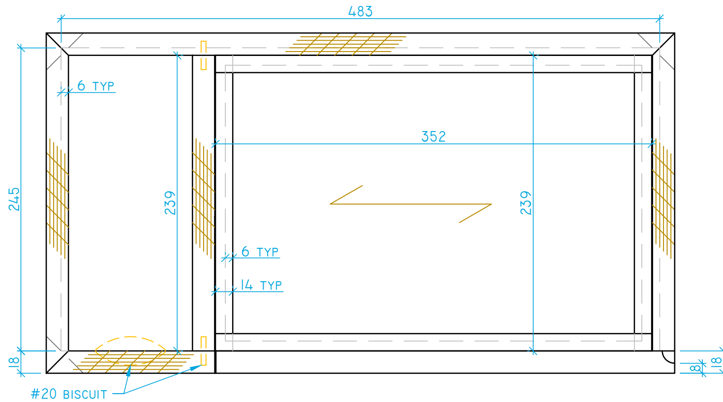
SECTION A : A SCALE 1 : 3
