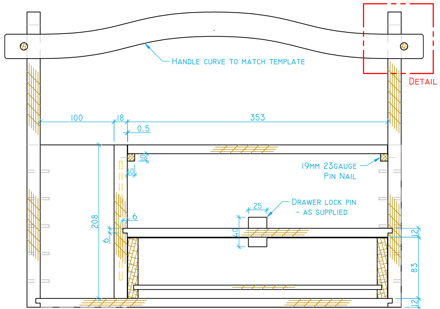
SECTION B : B SCALE 1 : 3
